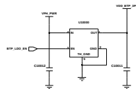
FOD LDO
